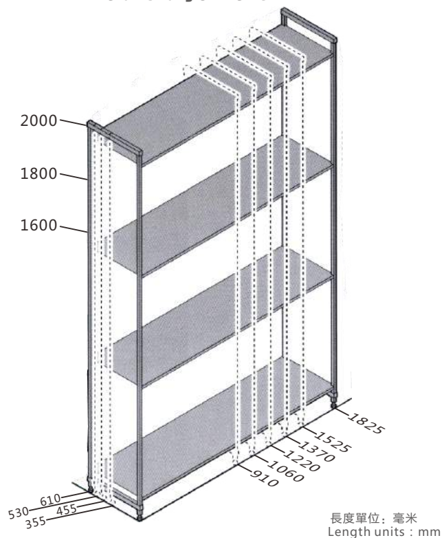
固定式架體尺寸 Stationary Unit Size
