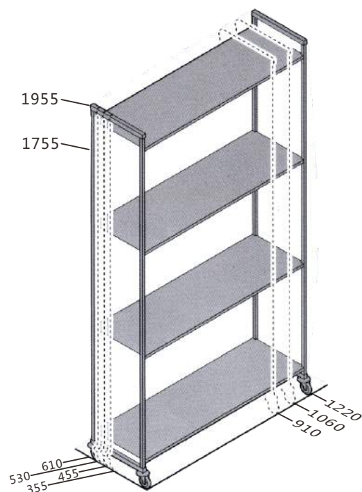
移動式架體尺寸 Mobile Unit Size
