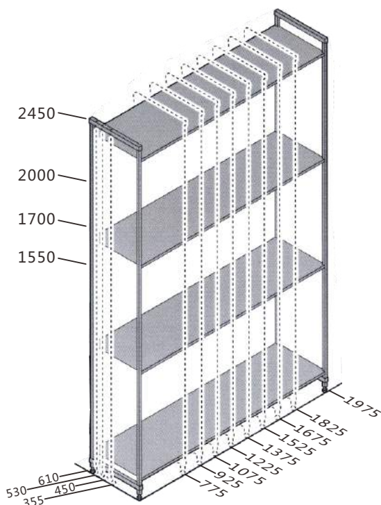
固定式架體尺寸 Stationary Unit Size
